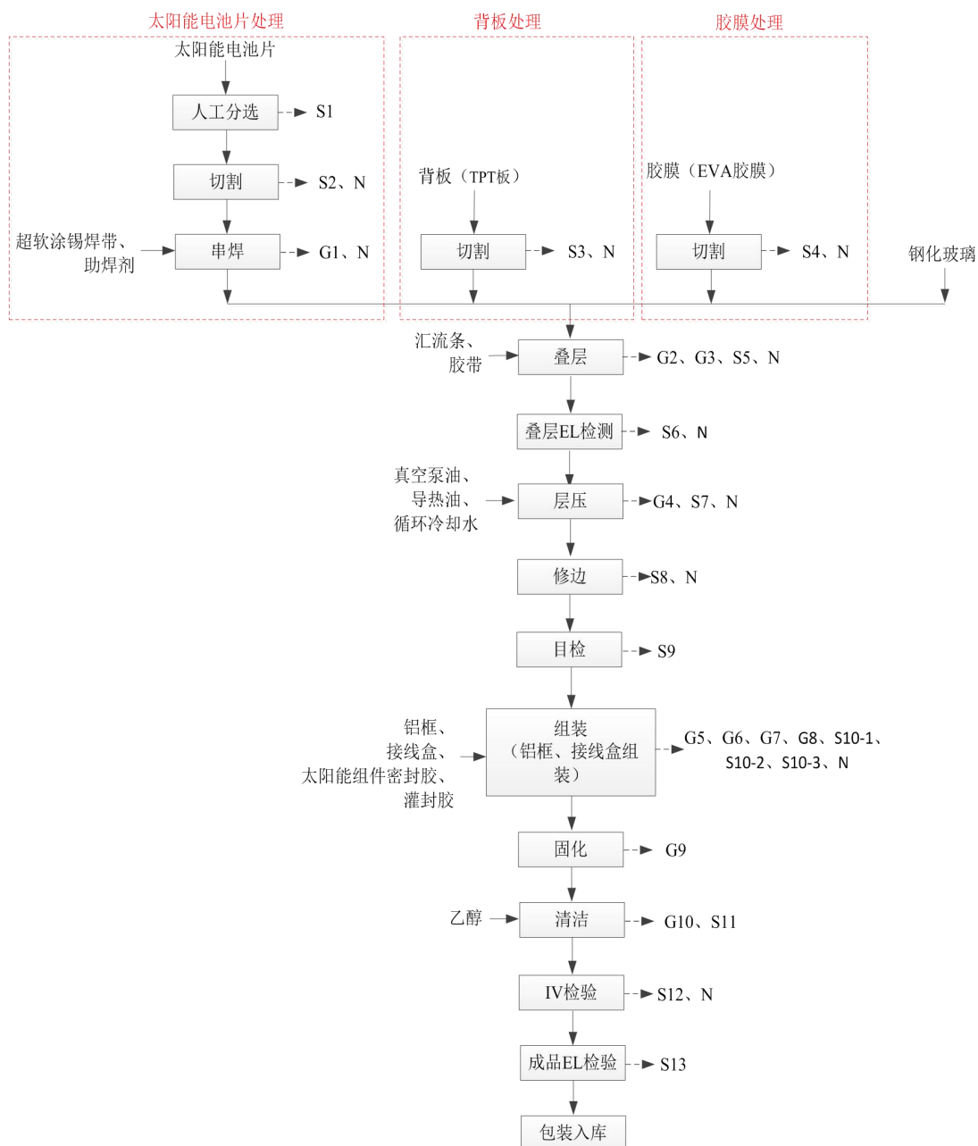
图 2-5 本项目生产工艺流程图
