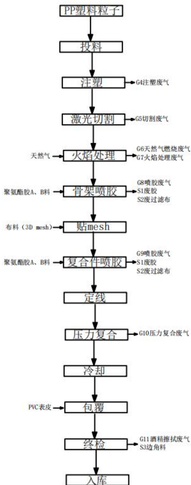
图 2-4 上盖板骨架生产工艺流程图
