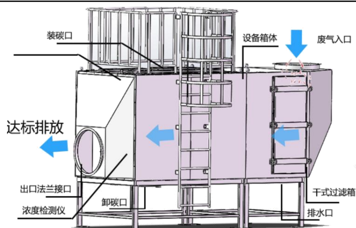
图 4-2 活性炭箱结构示意图
