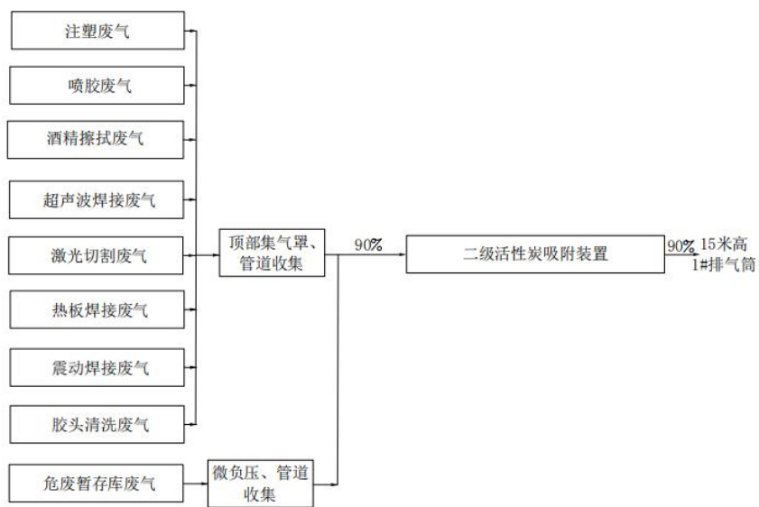
图 4-1 废气处理工艺示意图
