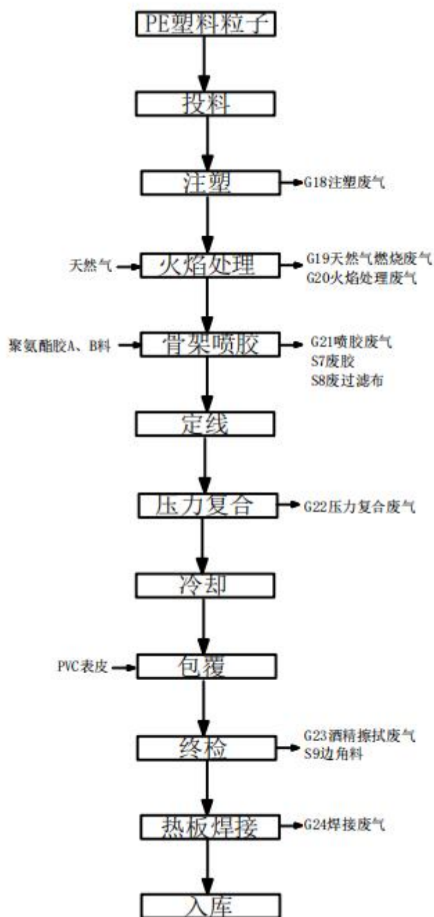
图 2-6 外板骨架生产工艺流程图
