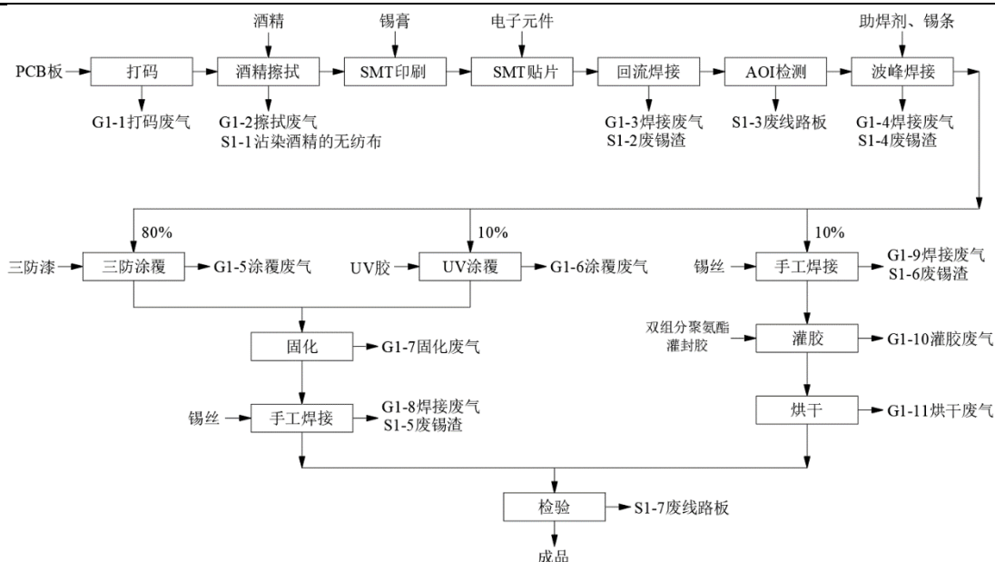
图 2-1 电机控制板生产工艺流程图
